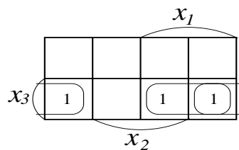
図 5: f のカルノー図
