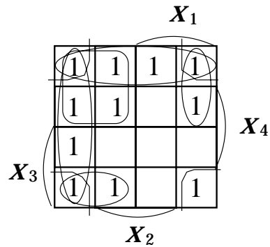
図 1: 4 変数のカルノー図
