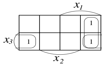
図 6: g のカルノー図
