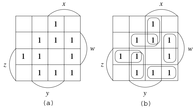
図 2: カルノー図
