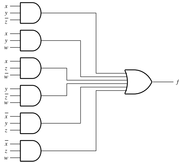
図 3: AND-OR 二段回路
