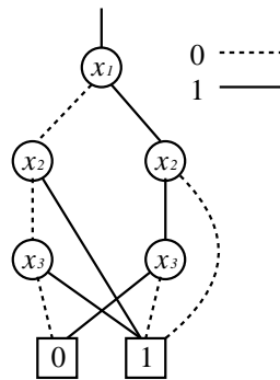
図 8: 5.48 の BDD
